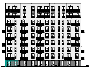
elevacja południowa
