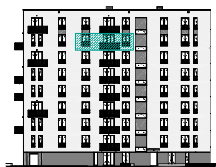
elewacja północna
